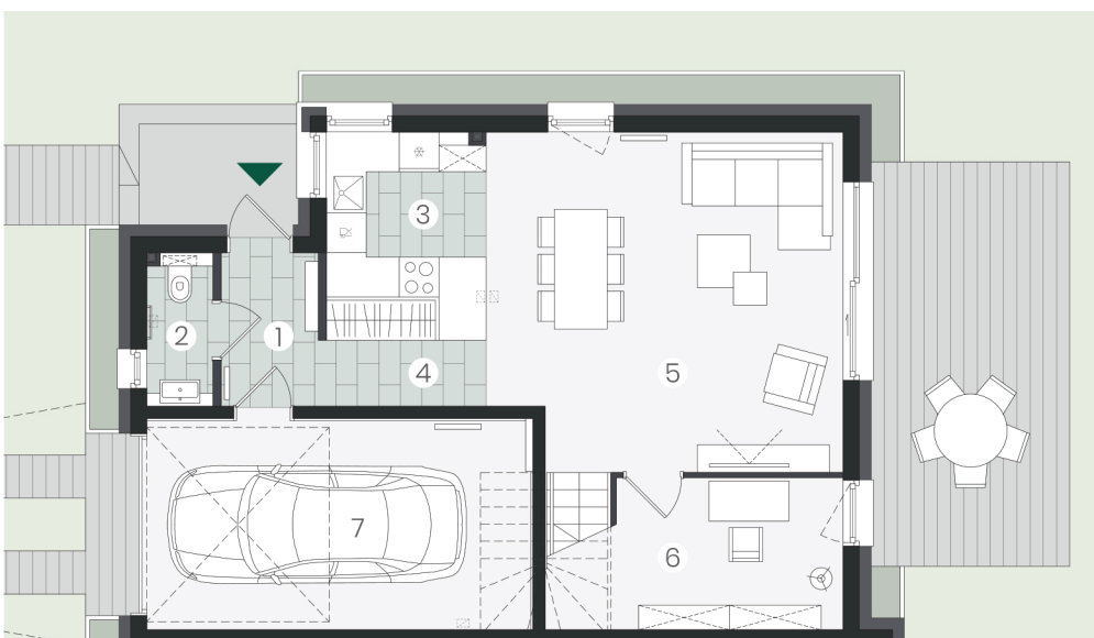
PARTER OPCJA 2 67,10m 2
